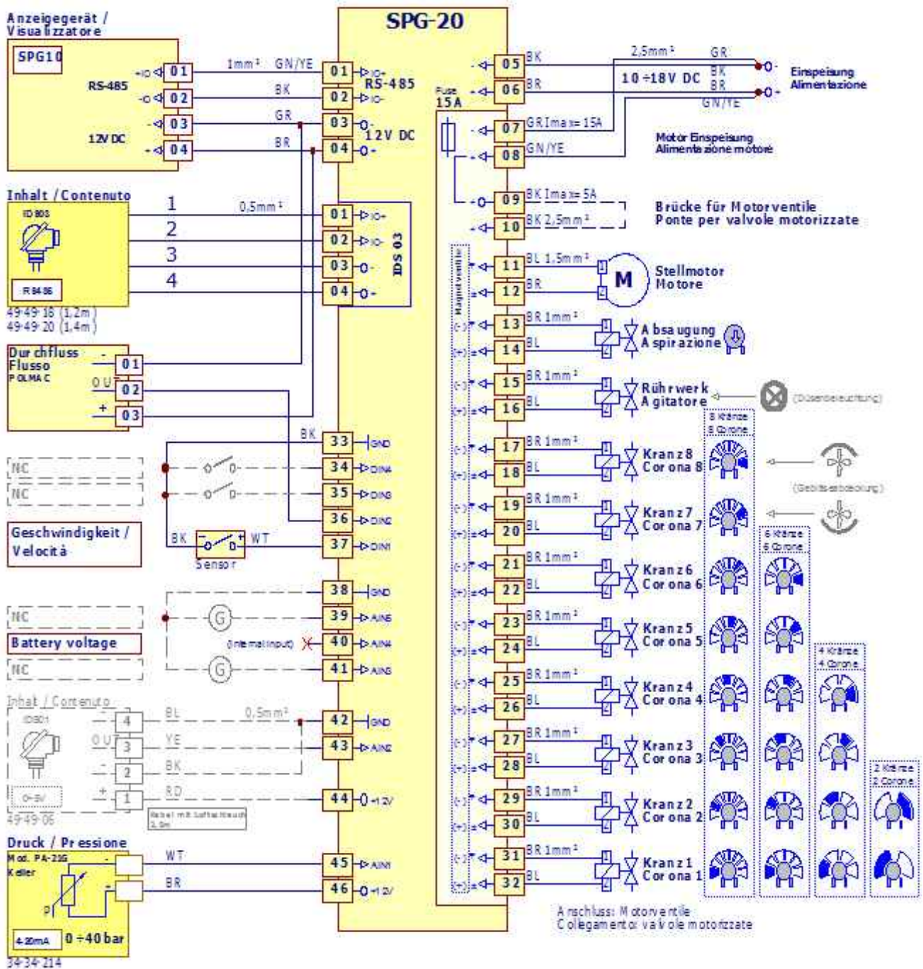
Abb. 44: Anschlussschema SPG20
