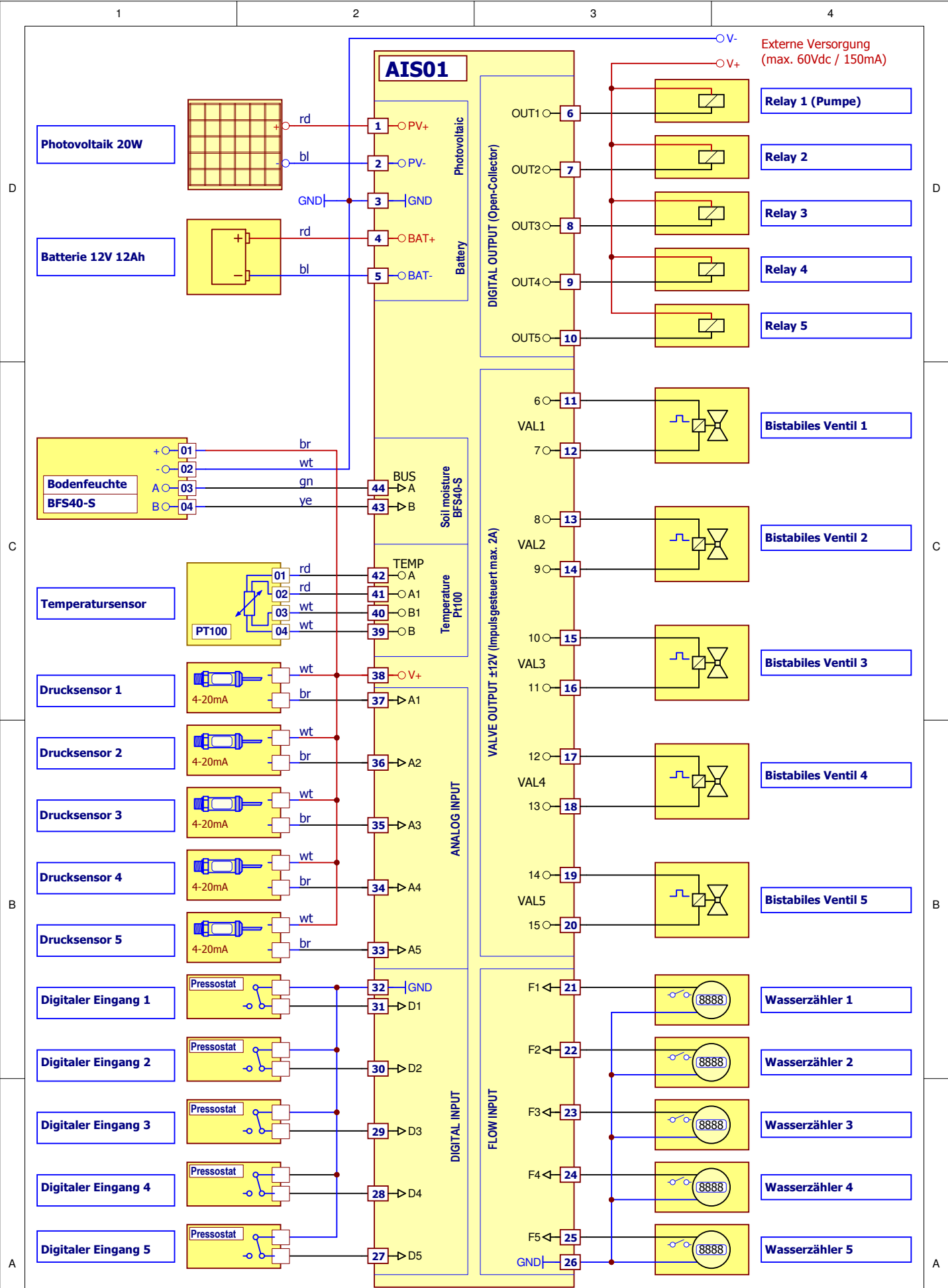
48-48-256 - AIS01 mit Bistabile Ventile - Anschlusschema Solar
